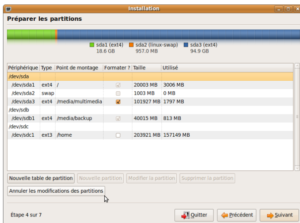
FIG. 2.10 – Sélection des disques durs et partitions
